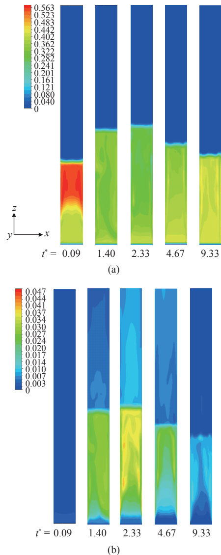
图 8 含水合物分解的气液固三相流动: (a) 固相体积分数的瞬时分布云图和 (b) 气相体积分数的瞬时分布云图 [49]
