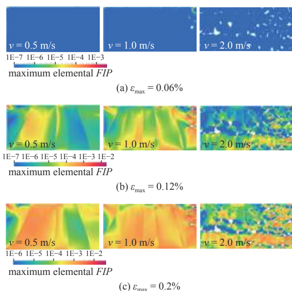
图6 x 方向不同应变幅 ( \epsilon_{\max} ) 下单元 FIP 分布
