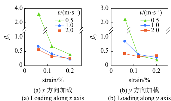
图 8 相对分散性参数 ( \beta_0/u_0 ) 变化曲线
