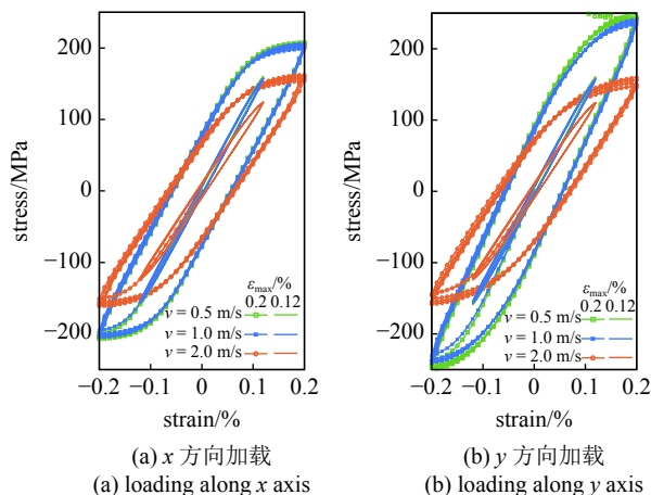
图5 不同应变幅 ( \epsilon_{\max} ) 下选区激光熔化增材制造微结构的循环应力-应变曲线
