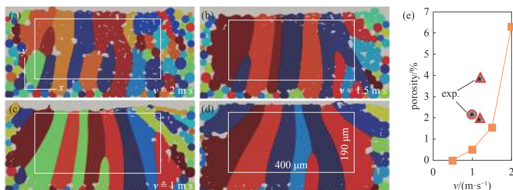
图 3 选区激光熔化增材制造微结构及其孔隙率: (a) v = 2 m/s; (b) v = 1.5 m/s; (c) v = 1 m/s; (d) v = 0.5 m/s; (e) 图 (a) ~ 图 (d) 中矩形区域 (400 \mu\text{m} \times 190 \mu\text{m} ) 的孔隙率, 其中圆形 (90 W, 1 m/s) [44] 和三角形 (160 W, 1.2 m/s) [45] 标记为实验结果
