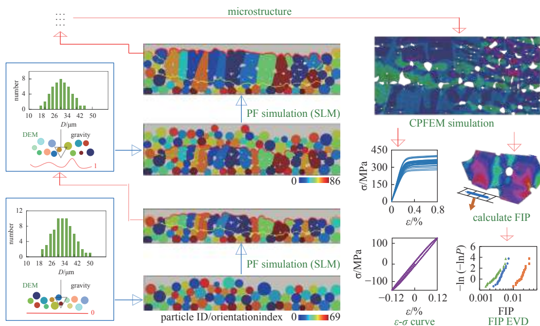
图1 用于增材制造微结构演化及疲劳分散性预测的集成离散元、相场模拟、晶体塑性有限元和极值概率理论的计算框架示意图 (DEM: 离散元; PF: 相场; CPFEM: 晶体塑性有限元; FIP: 疲劳指示参数; EVD: 极值分布)
