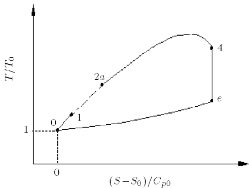
图 2 PDE 工质热循环温熵图
