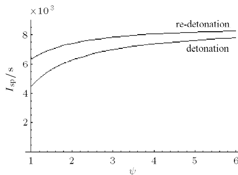
图 11 多级重复起爆 PDE 工质比冲 (基于燃料)
