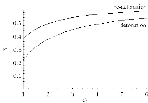
图 10 MPRDE 工质热循环效率
