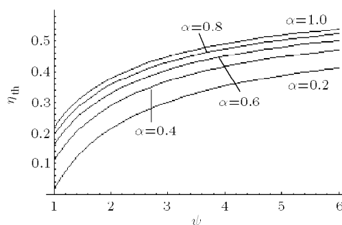
图 3 总压恢复系数 \alpha 对热循环效率 \eta_{th} 的影响
