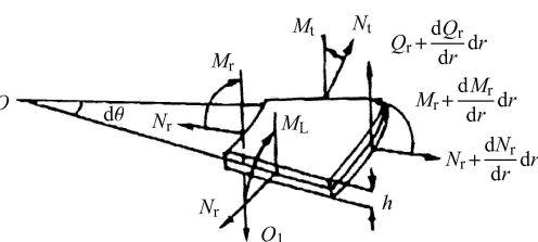
(b) 基于 Kirchhoff 经典薄板理论的筛板力学模型 [54]
