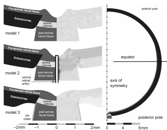
图 13 视乳头区域有限元计算模型 [67]
