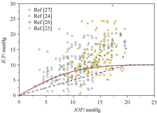
图 2 IOP 与 ICP 的关系. 其中, 虚线与实线分别表示由式 (1) 与式 (2) 得到的理论结果, 实验数据 [24-27] 则由不同的符号表示 Fig.2 The relations between IOP and ICP. The broken line stands for Eq.(1), the solid line expresses Eq.(2), and different figurate points indicate the different experimental data from Refs.[24-27]
