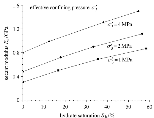
图 3 不同有效围压下水合物沉积物割线模量随水合物饱和度变化曲线
